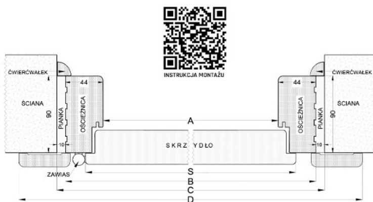
WYMIARY SKRZYDŁA I OŚCIEŻNICY STAŁEJ
