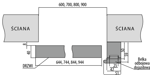
Rysunek systemu przesuwnego ściennego bez zabudowy
