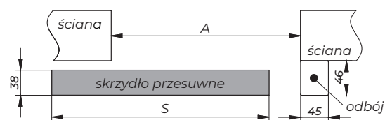
szerokość systemów podwójnych naściennych
