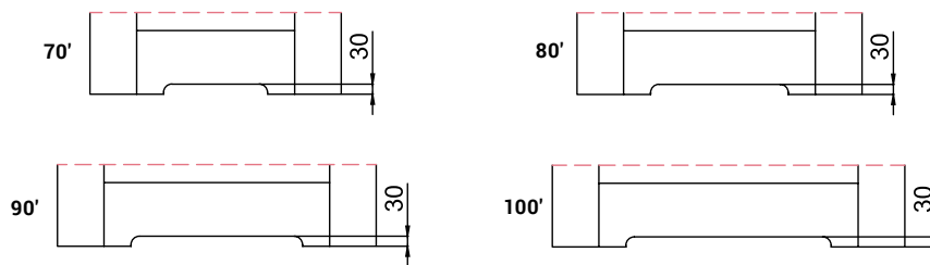
WIELKOŚĆ PODCIĘCIA WENTYLACYJNEGO W DRZWIACH RAMOWYCH **)
