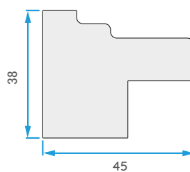
Profil listwy
