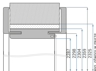
Wymiary ościeznica do drzwi PN23
