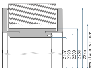
Wymiary ościeznica do drzwi PN22
